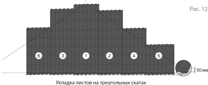
Укладка листов на треугольных скатах
