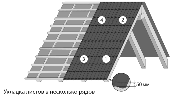
Укладка листов в несколько рядов
